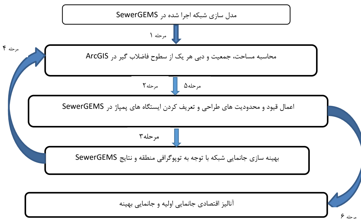
شکل ۱. فلوچارت مراحل بهینه سازی و اصلاح شبکه
