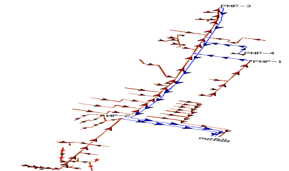
شکل ۲. جهت جریان و محل قرارگیری پمپ‌ها و خروجی‌ها در طرح اجرا شده قدیمی
